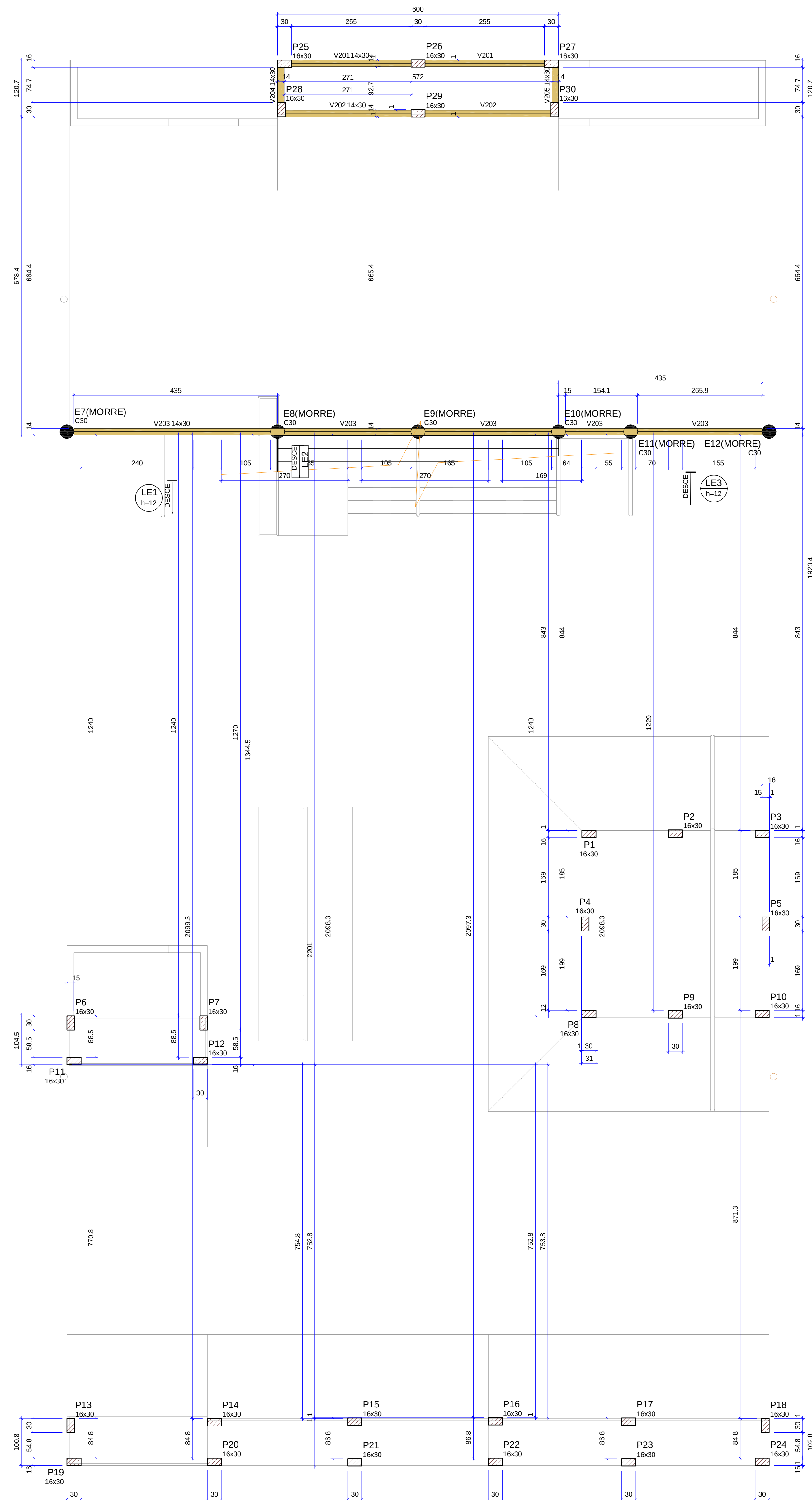
Forma do pavimento Base superior (Nível 100)
